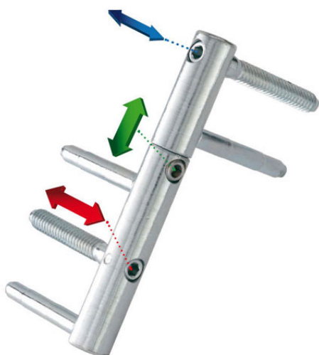
REGULACJA BOCZNA W SKRZYDLE
